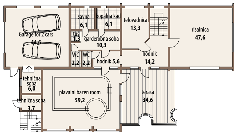
1 nadstropje 282,6 m 2
