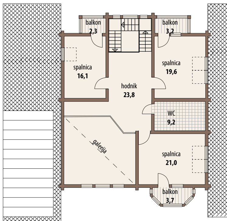
2. nadstropje 110,8 m 2
